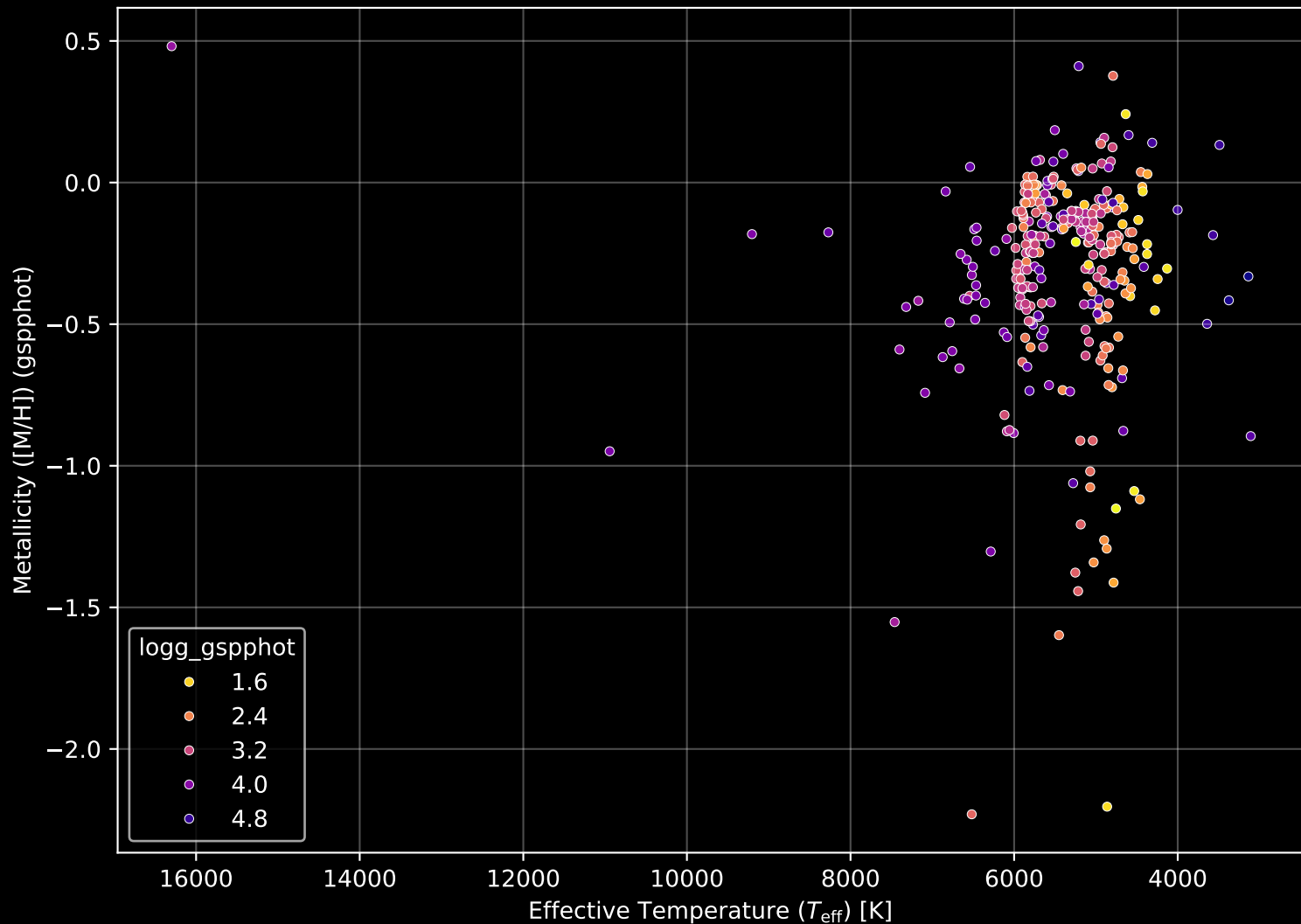
APOGEE DR17 Field: [M13] Stellar Population Parameters (n= 333)
